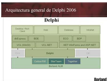
Figura 2: Arquitectura general de Delphi 2006
