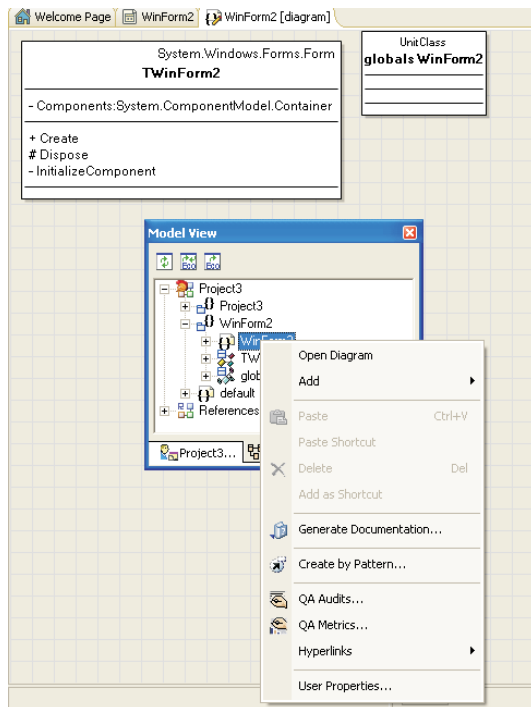
Figura 3: Opciones de Together en Delphi 2006
