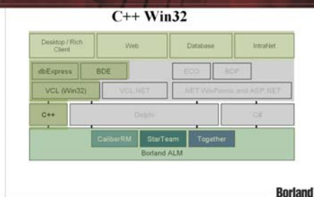
Figura 4: Arquitectura general de C++ Win32
